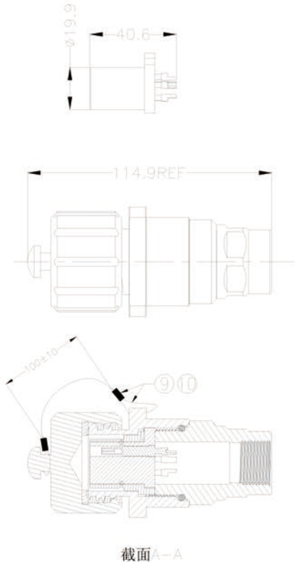
截面A-A
